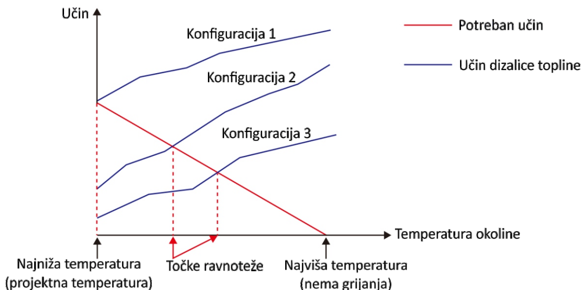
Slika 1-1.1: Konfiguracija sustava
